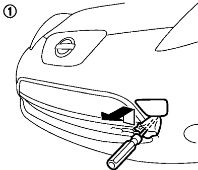
Avant
